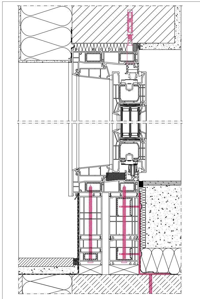
rys 5. Przekrój pionowy
