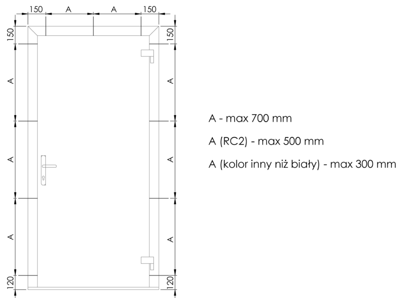
Rys. 2 Rozmieszczenie punktów mocujących
