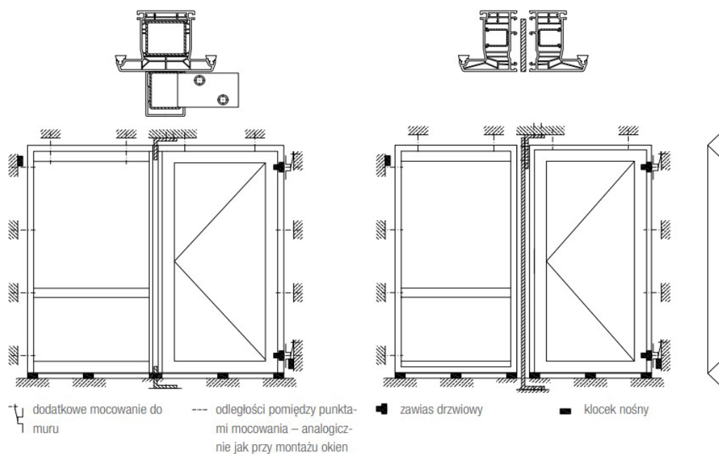
Rys. 4 Montaż zestawu drzwi zewnętrznych
