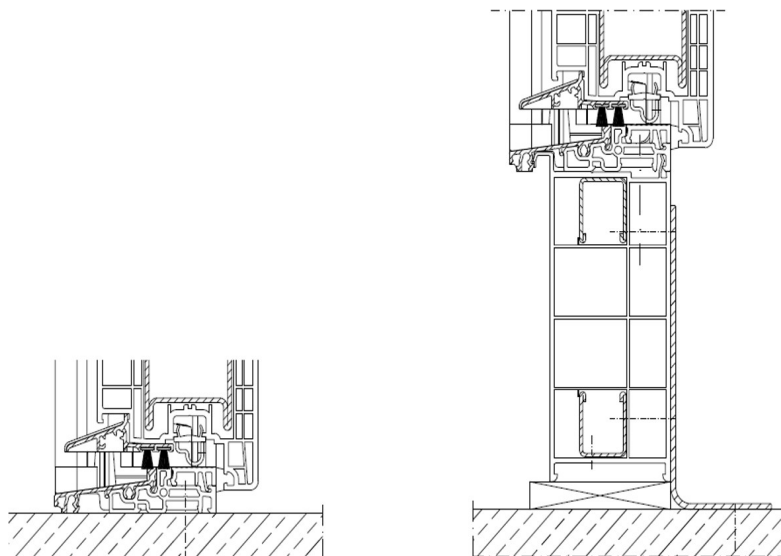
Rys. 3 Montaż progu (bezpośrednio do posadzki oraz do poszerzenia)
