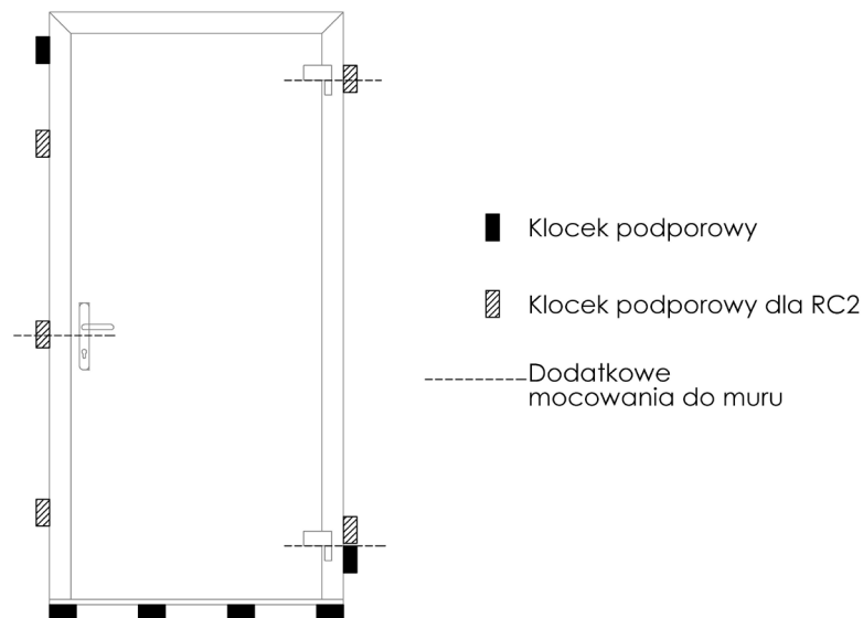
Rys. 1 Sposób podparcia drzwi PVC
